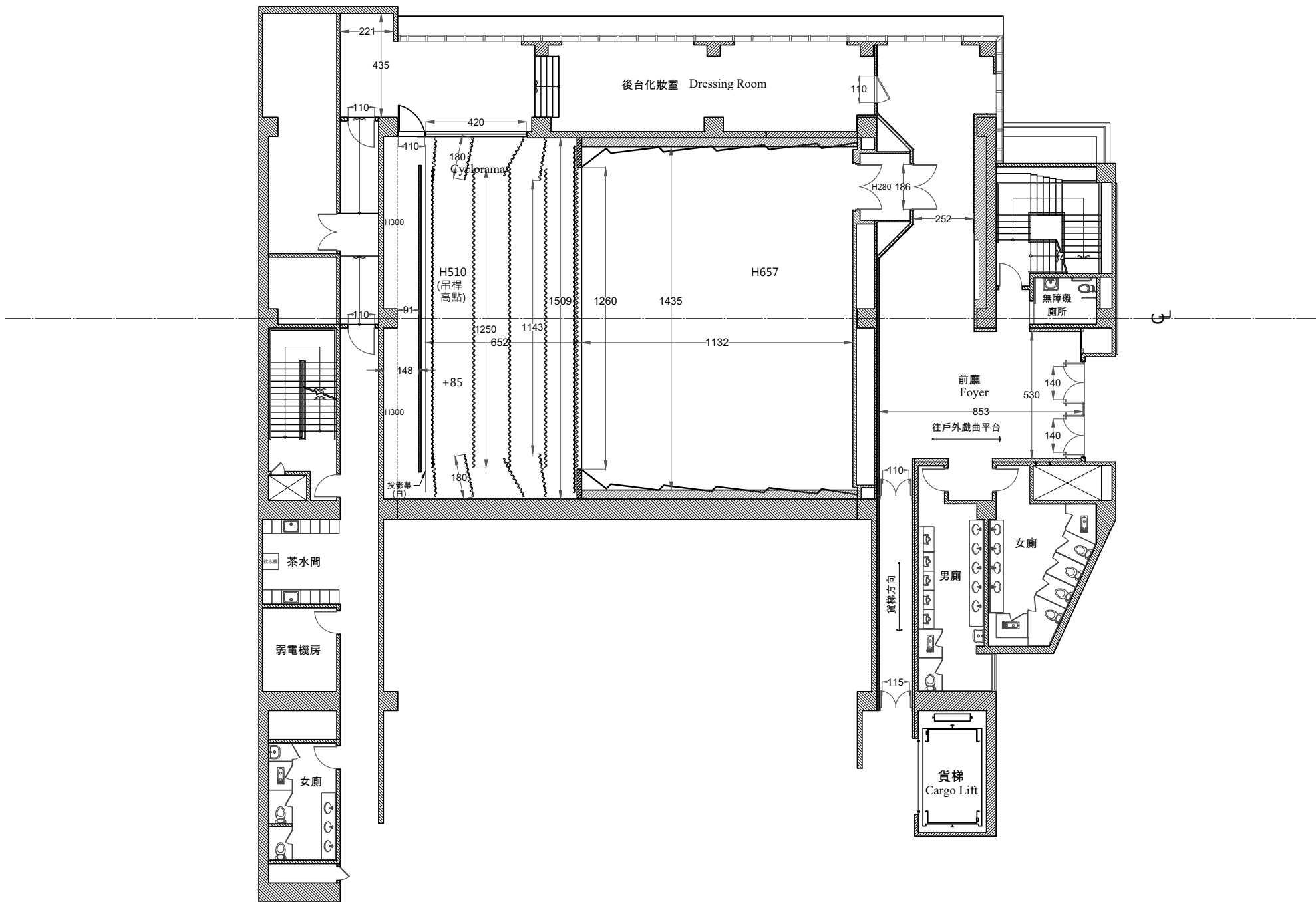
圖 (一) 小舞台(3201)_平面圖 (單位：公分) Figure(1) Small Stage(3201)_Floor Plan (Unit: cm)
